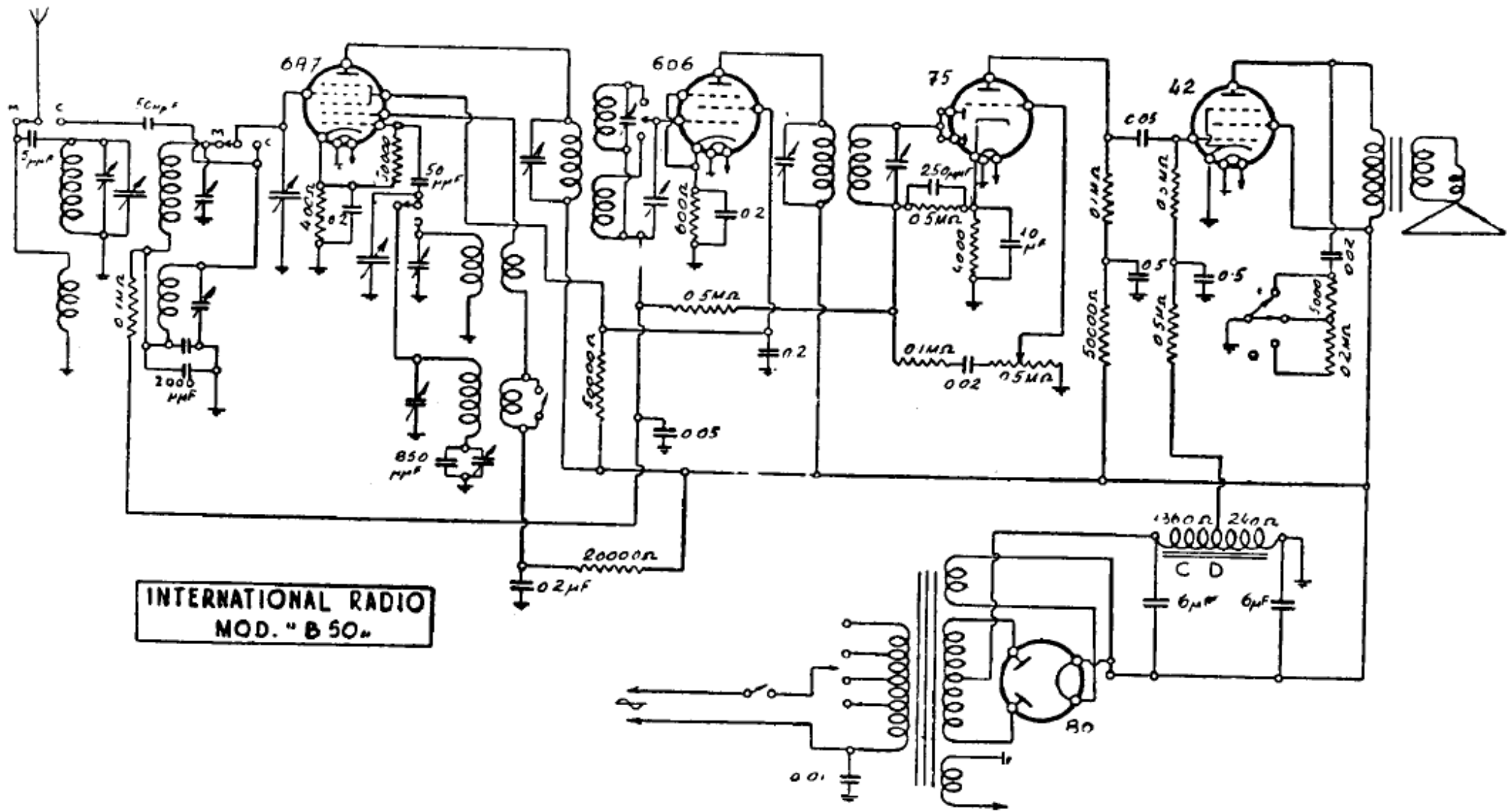
IRRADIO. — Modello « B 50 » Produzione '935 Media frequenza: 250 kc.
